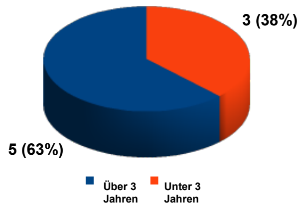
Mit Wirbelsäulenerkrankung nach Altersklassen
